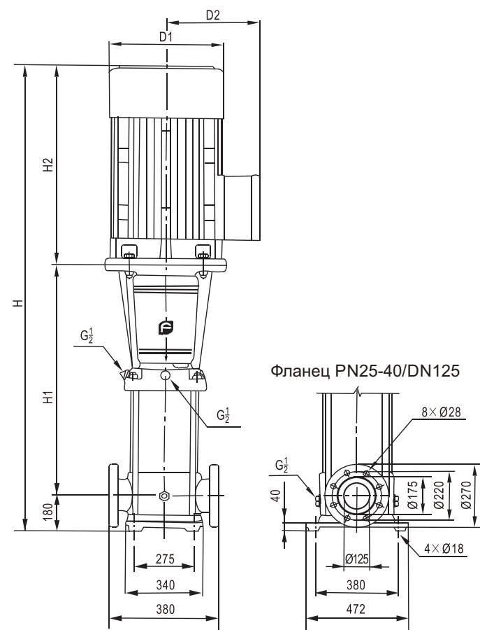
Габаритно-присоединительные размеры однофазного электродвигателя и взрывозащищенного двигателя имеют небольшие отличия. Пожалуйста, обратитесь в представительство в вашем регионе для уточнения.
